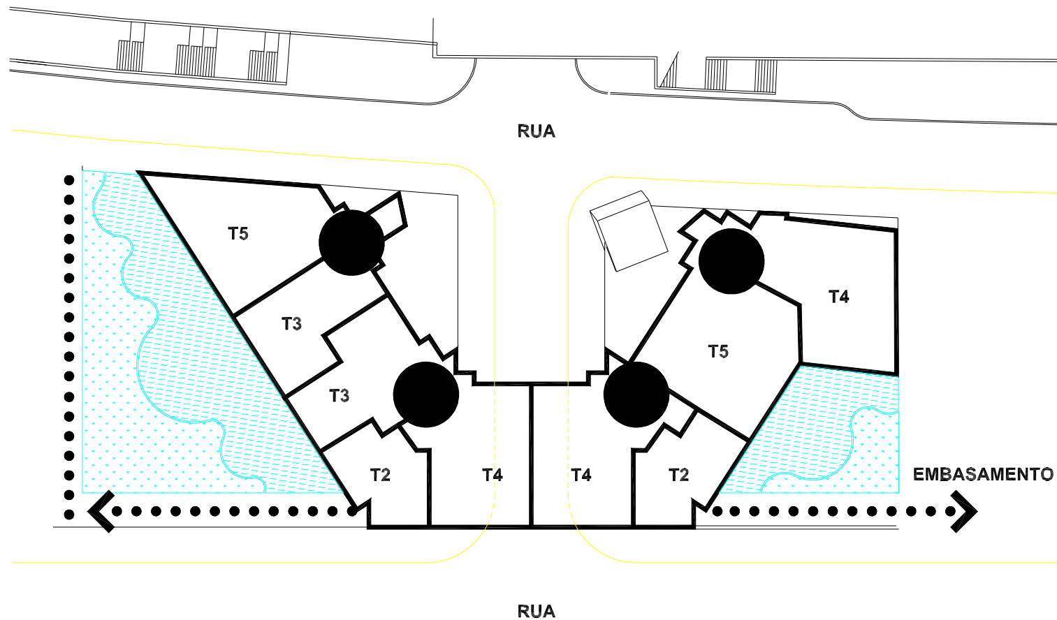
PLANTA PISOS 0-12
