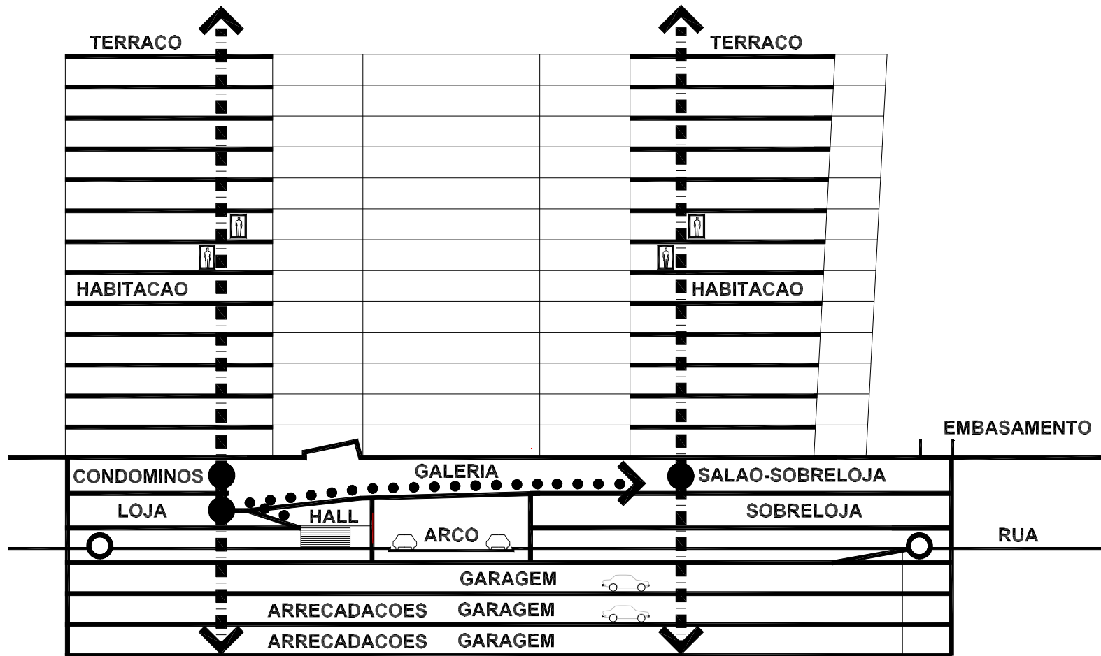
CORTE LONGITUDINAL
